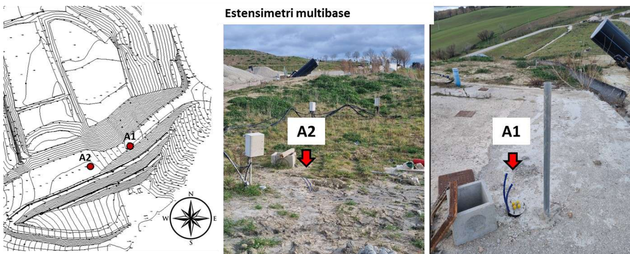
Figura 52 – Posizione delle verticali estensimetriche
