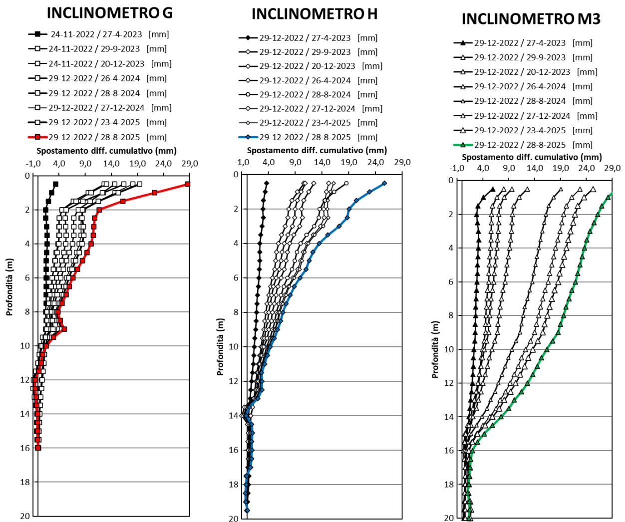
Figura 29 – Inclinometri G (zero al 24-11-2022), H (zero al 29-12-2022) e M13 (zero al 29-12-2022): deformata differenziale integrale dal basso per quadrimestri successivi
