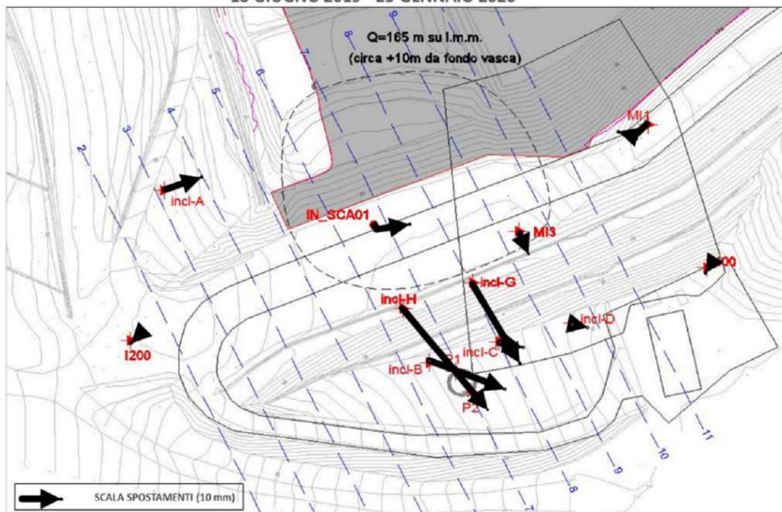
Figura 17 – Spostamenti inclinometrici GEN - GIU 2019 e GIU 2019 – GEN 2020
