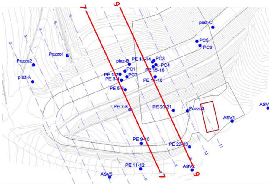
Figura 30 – Planimetria dell'argine con indicazione delle verticali di monitoraggio piezometrico
