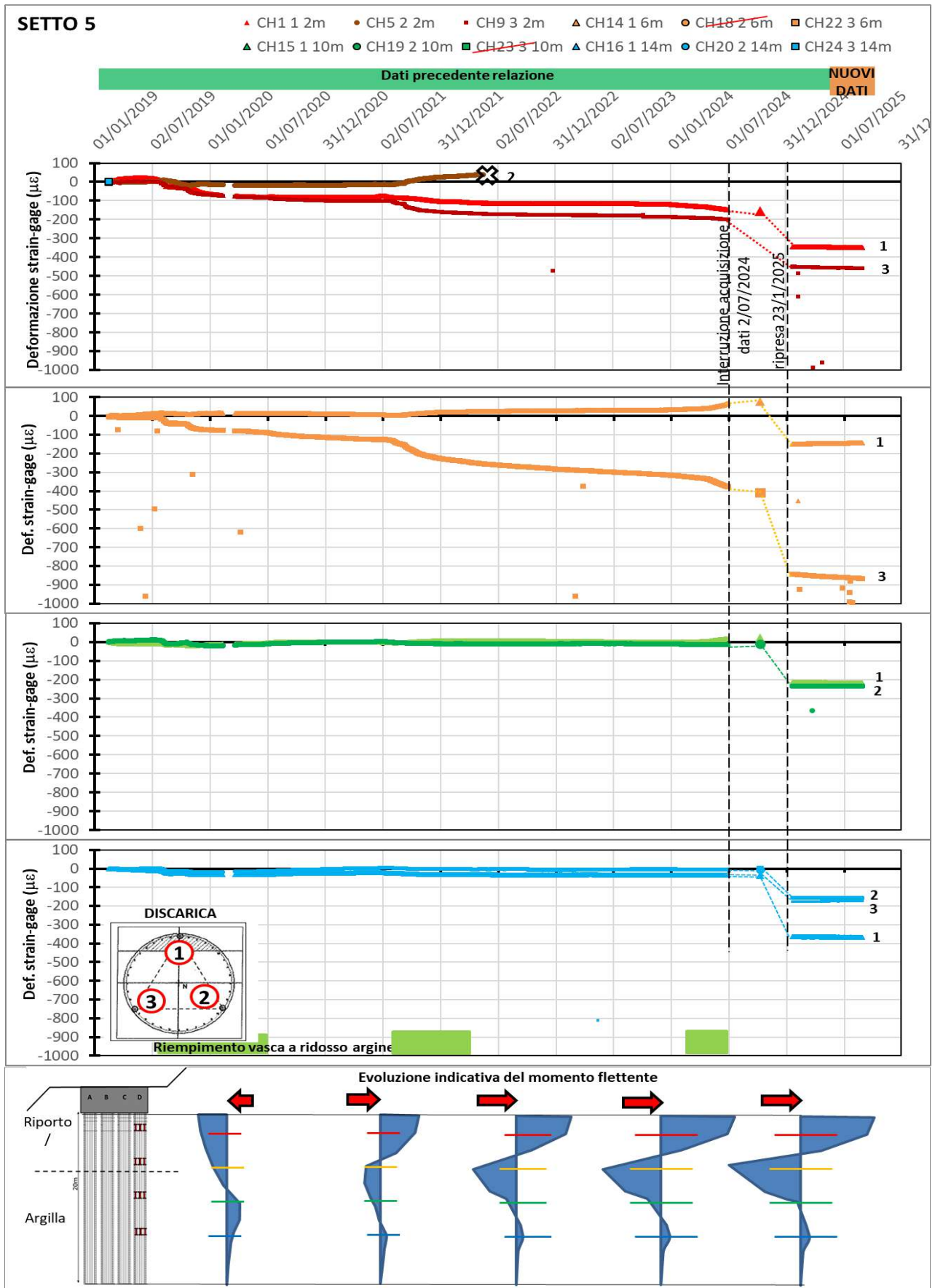
Figura 48 – Andamento temporale della lettura agli strain-gages del palo D su setto n.5
