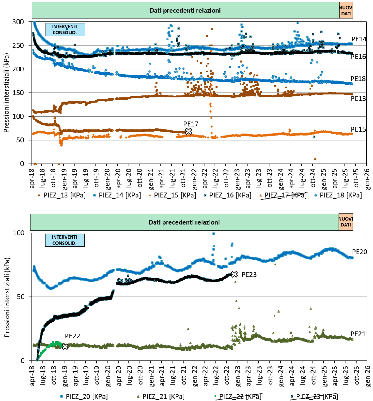
Figura 33 – Andamento nel tempo delle pressioni interstiziali misurate dalle celle PE13-PE23
