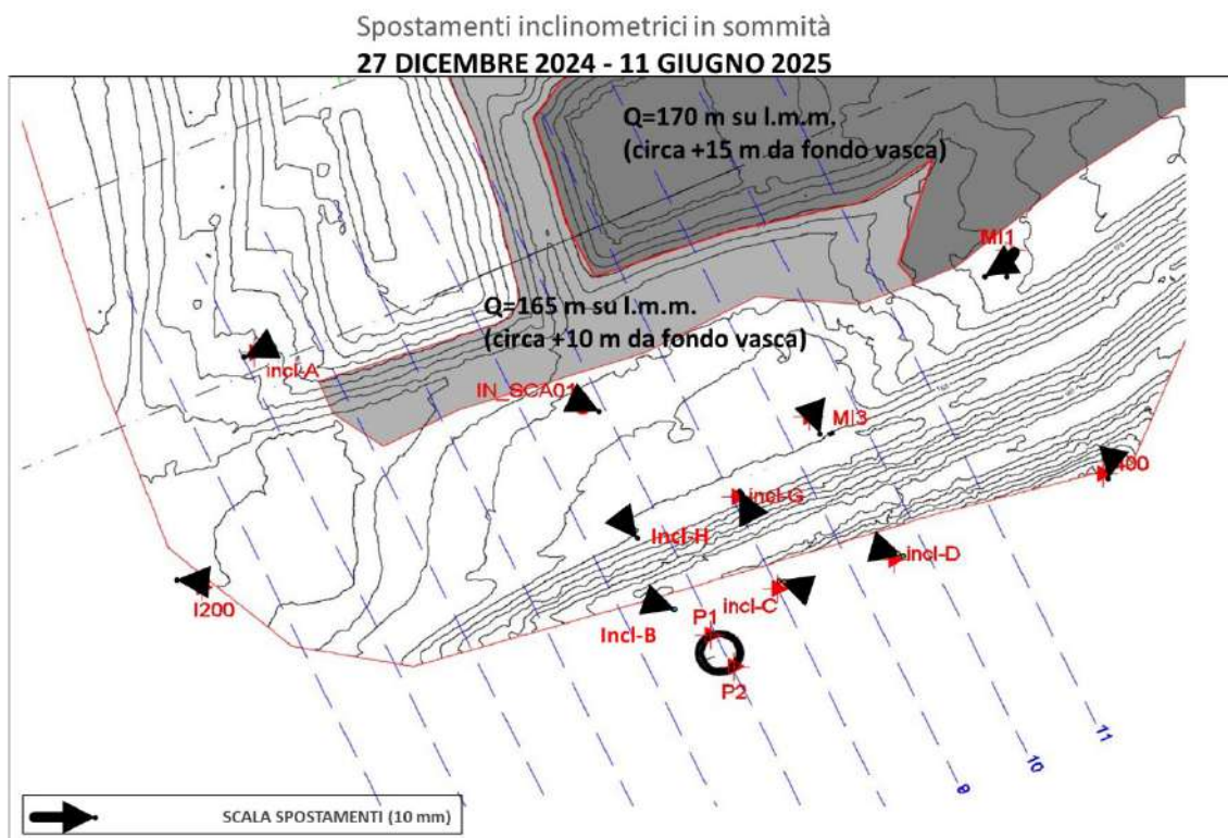
Figura 23 – Spostamenti inclinometrici DIC 2024 – GIU 2025
