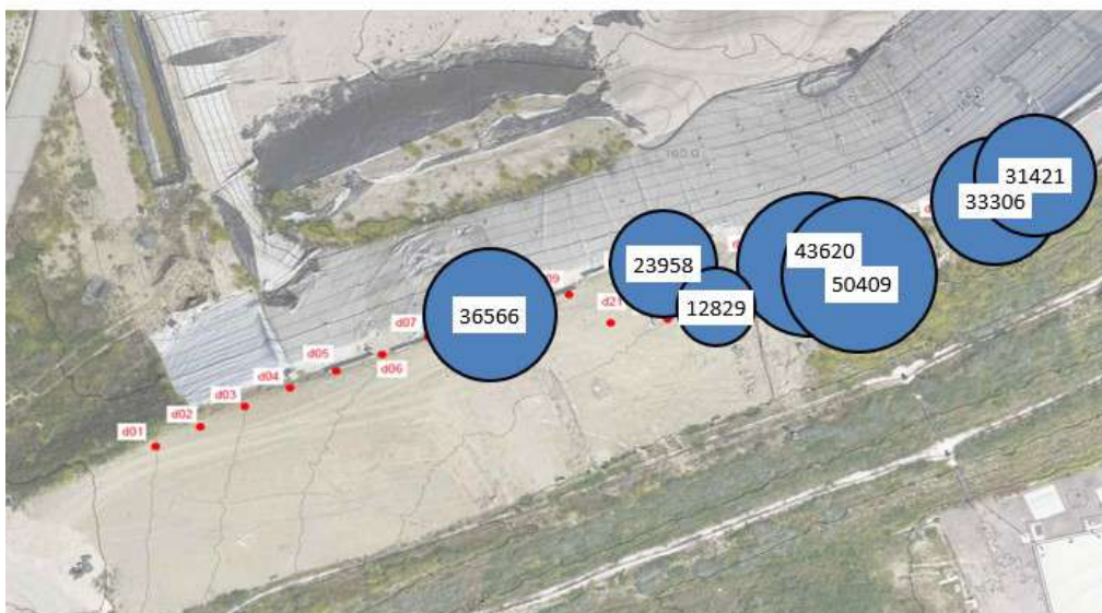
Figura 39 – Rappresentazione grafica delle portate emunte nel periodo OTTOBRE 2019–AGOSTO 2025
