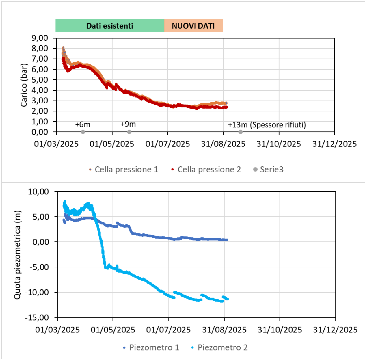
Figura 56 – Misure alle calle di carico totale e ai piezometri elettrici
