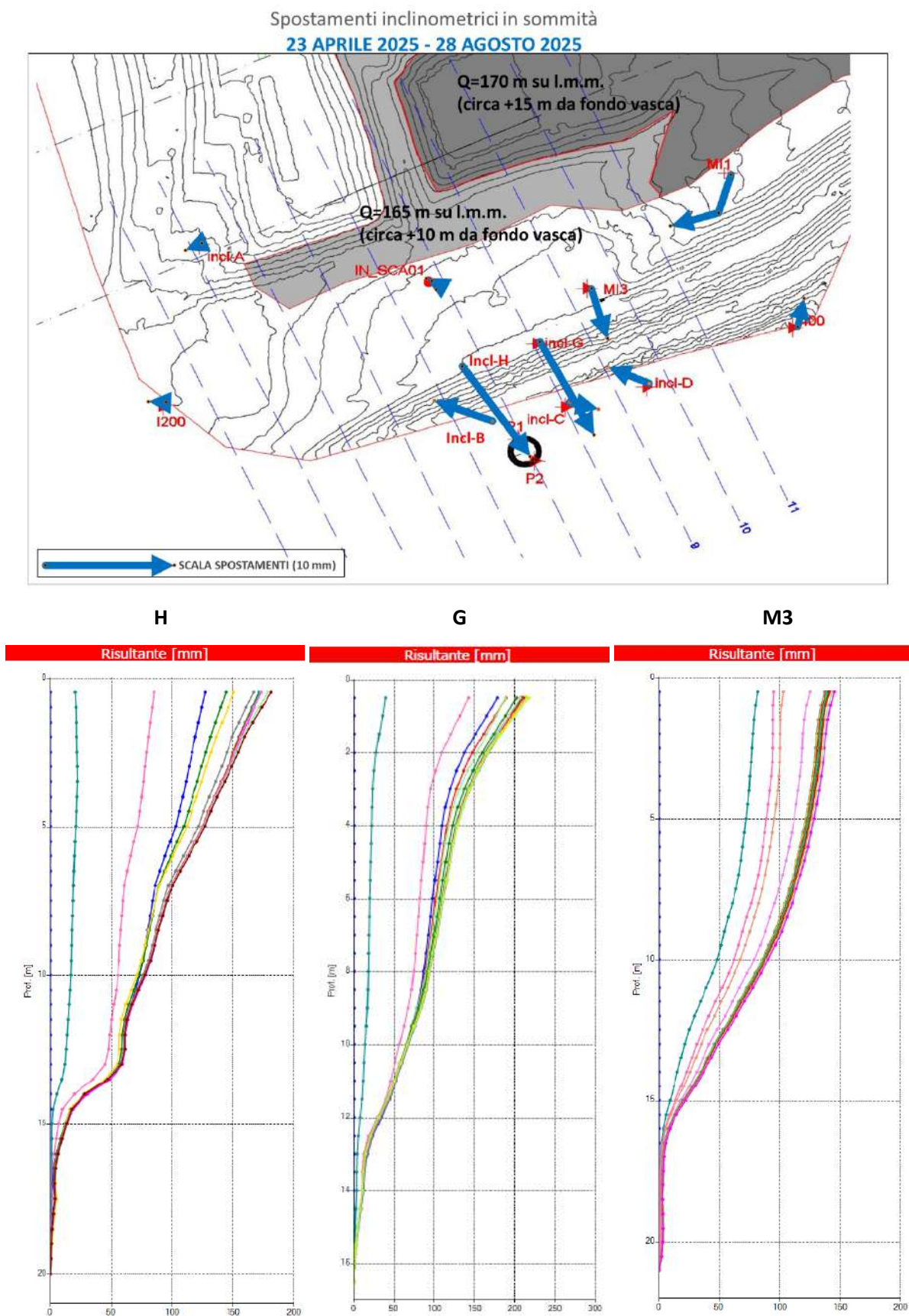
Figura 24 – Spostamenti inclinometrici APR – AGO 2025 (in scala di rappresentazione amplificata) e deformate inclinometriche complessive delle verticali H, G, M3
