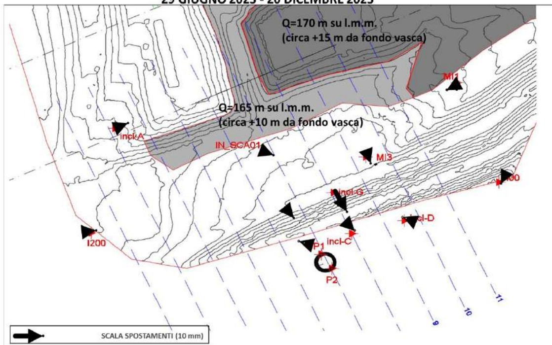
Figura 21 – Spostamenti inclinometrici DIC 2022 – GIU 2023 e GIU - DIC 2023
