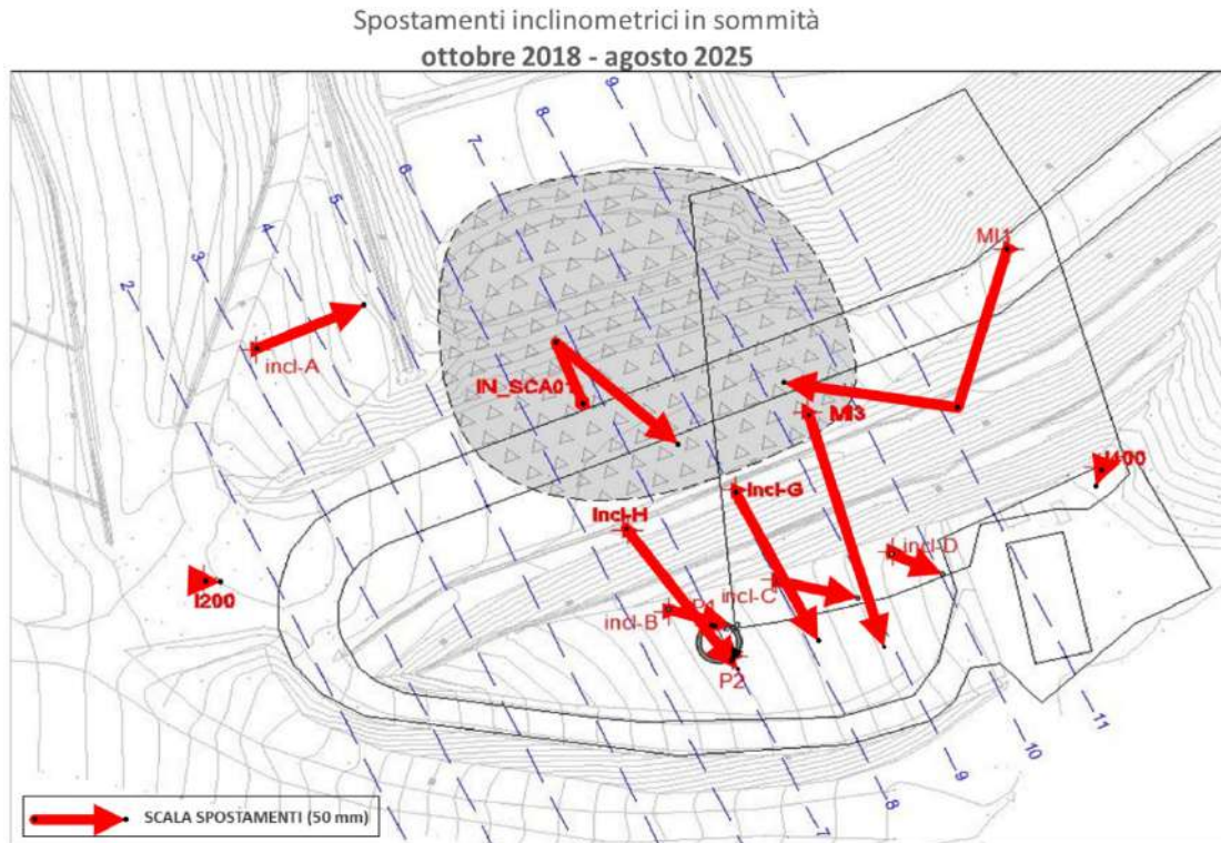
Figura 16 – Spostamenti inclinometrici nel periodo OTTOBRE 2018 – AGOSTO 2025
