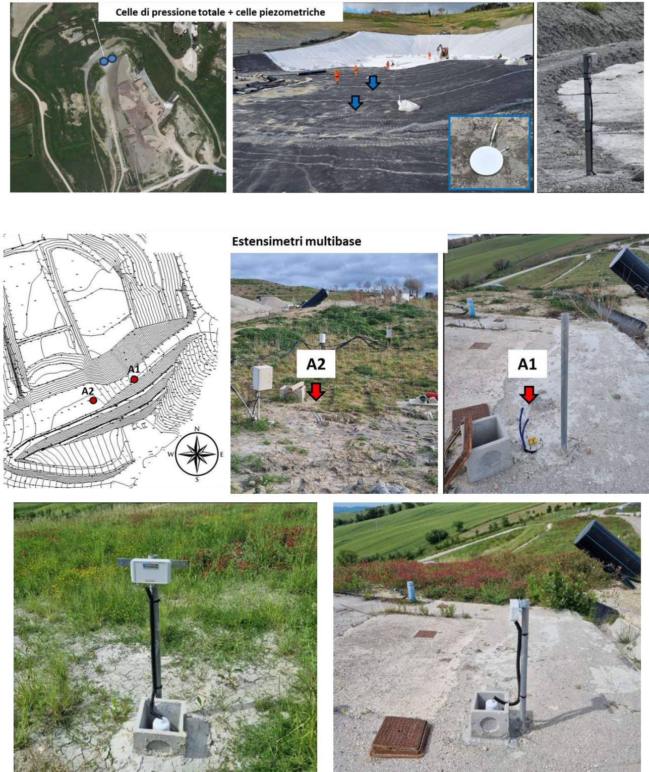
Figura 5 – Fotografie degli strumenti integrativi di monitoraggio installati
