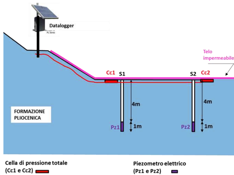
Figura 55 – Schema di installazione degli strumenti
