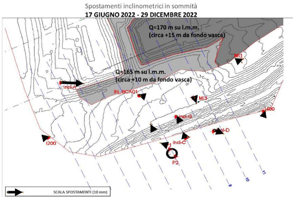
Figura 20 – Spostamenti inclinometrici GEN – GIU 2022 e GIU – DIC 2022
