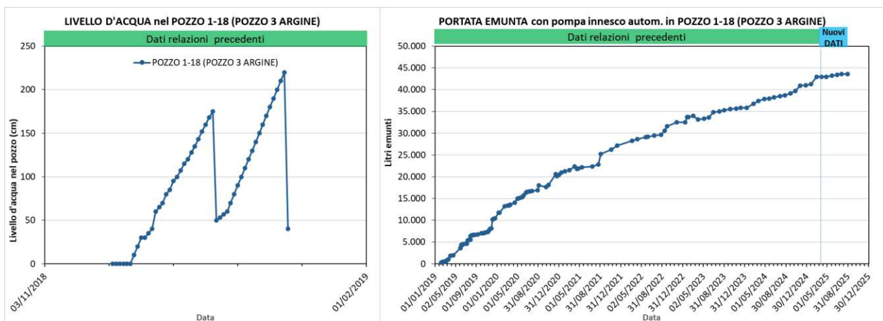
Figura 36 – Portata emunta dal POZZO 1-18 (fino ad AGOSTO 2025)
