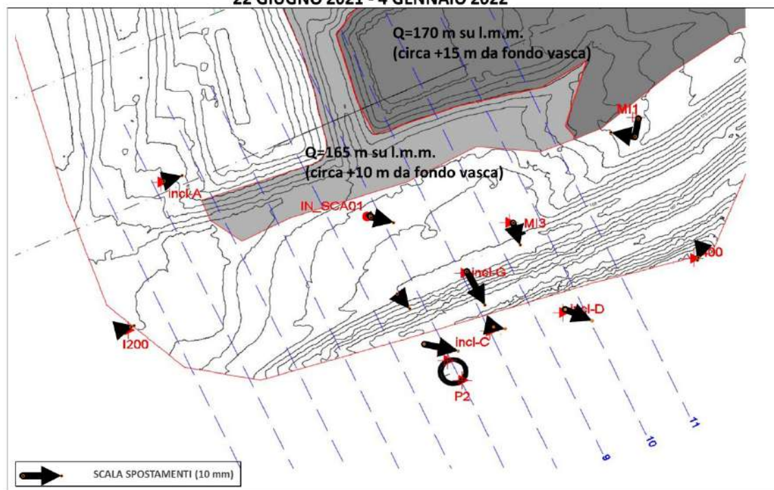
Figura 19 – Spostamenti inclinometrici GEN – GIU 2021 e GIU 2021 – GEN 2022
