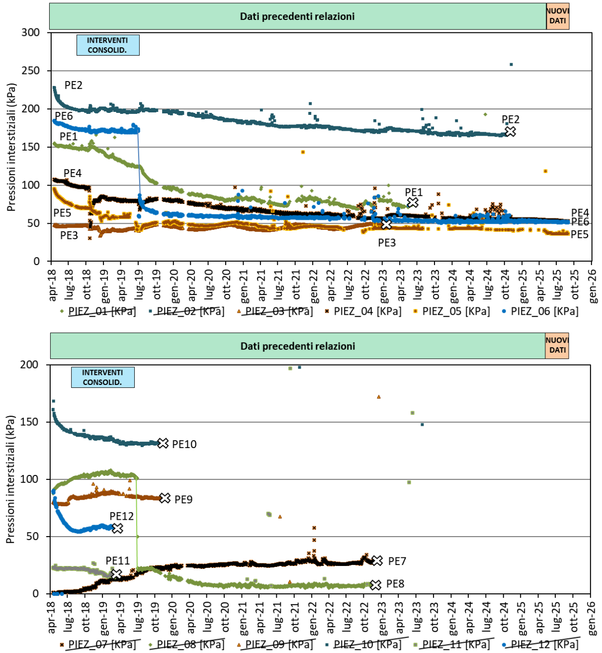
Figura 32 – Andamento nel tempo delle pressioni interstiziali misurate dalle celle PE1-PE12
