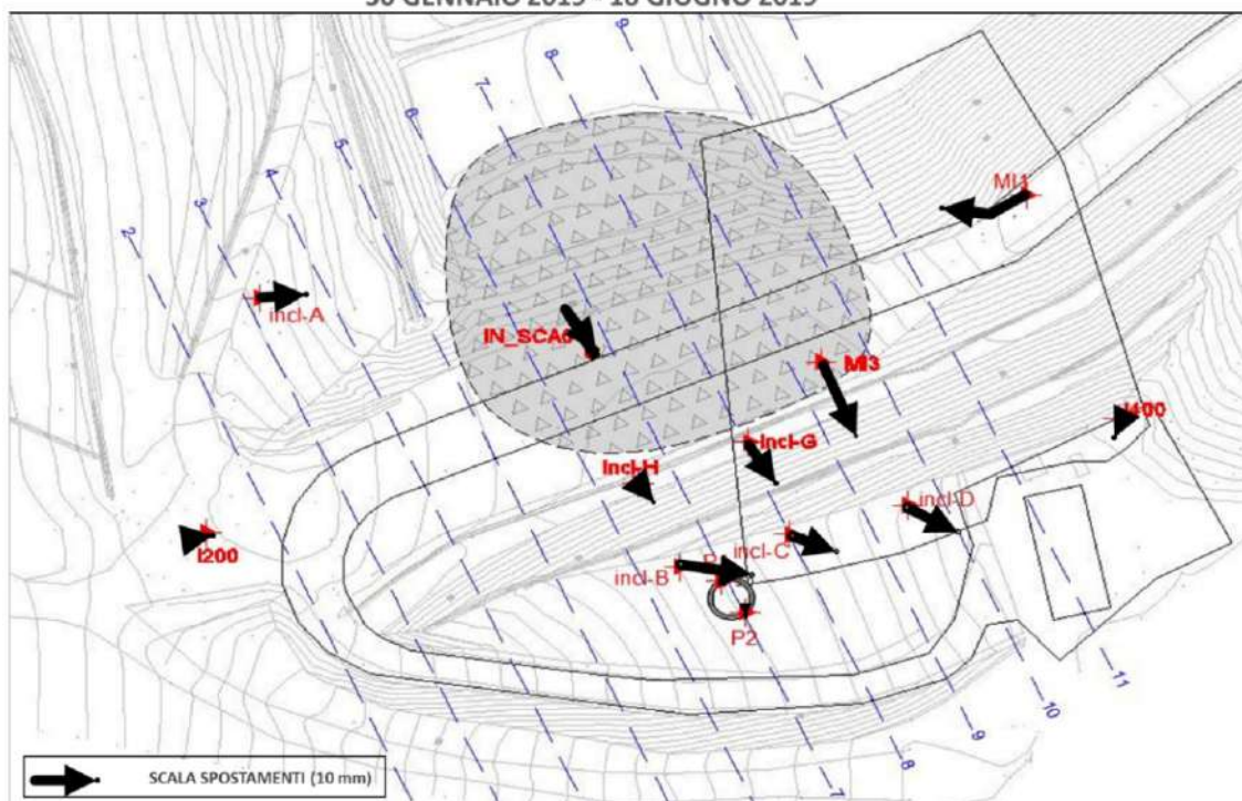
Spostamenti inclinometrici in sommità 18 GIUGNO 2019 - 23 GENNAIO 2020
