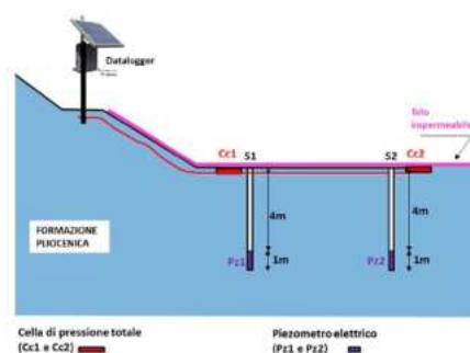
Figura 53 – Posizione delle celle di carico totale e dei piezometri
