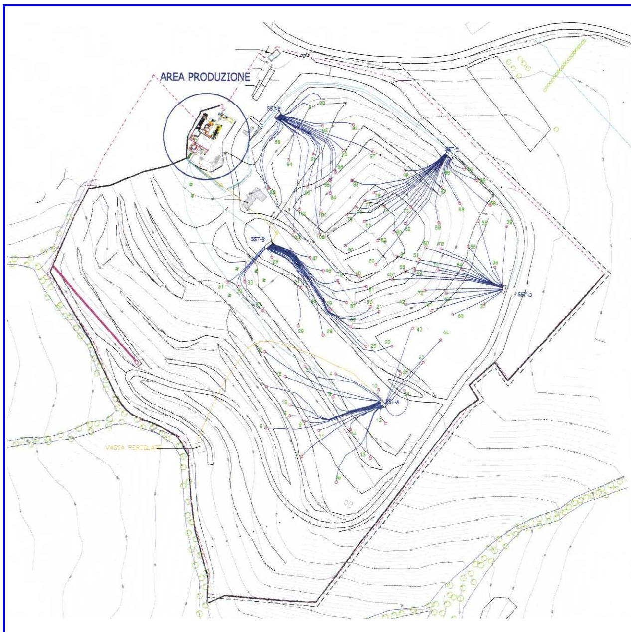
Planimetria ubicazione camini biogas
