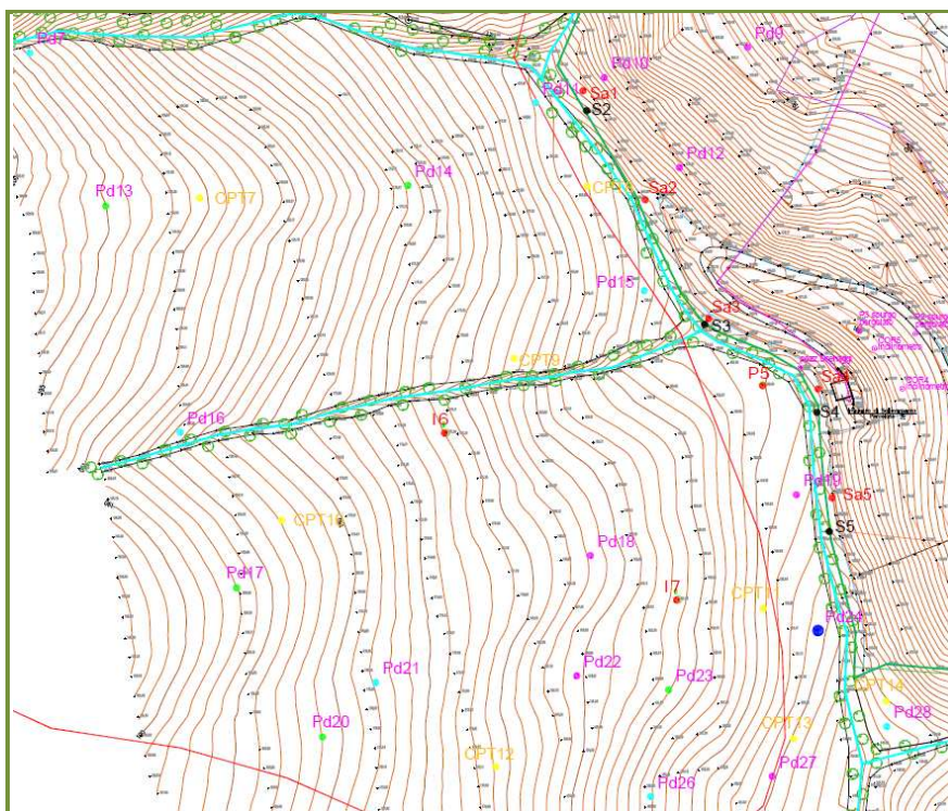
Individuazione piezometri esterni all'impianto di smaltimento PD21÷PD7
