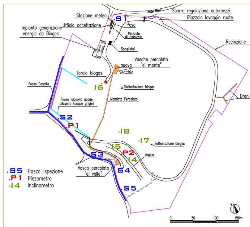
Ubicazione strumentazioni
