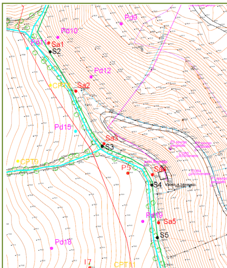
Individuazione pozzi/piezometri Sa1÷Sa5
