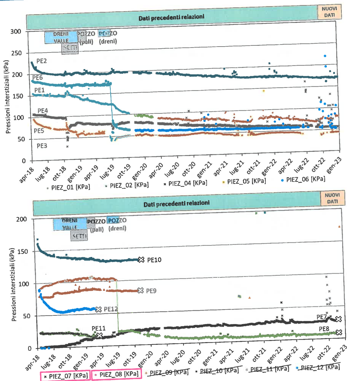
Figura 24 – Andamento nel tempo delle pressioni interstiziali misurate dalle celle PE1-PE12
