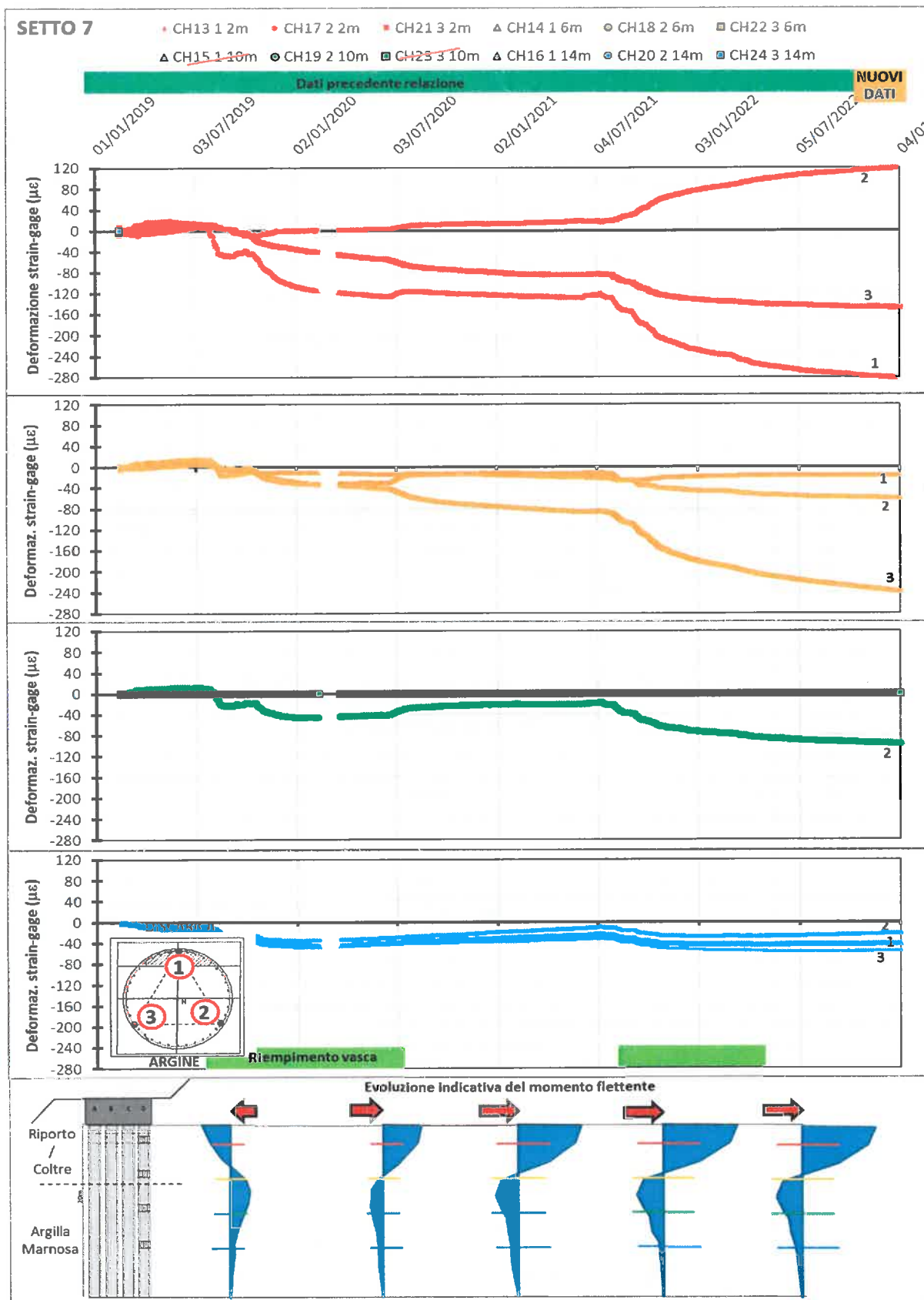
Figura 41 – Andamento temporale della lettura agli strain-gages del palo D su setto n.7
