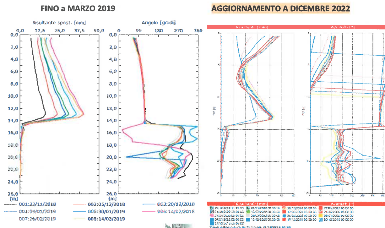
Figura 18 – Inclinometro SCA01 (zero al 31-10-2018): deformata differenziale integrale dal basso e azimut nel periodo iniziale con il dissesto interno attivo (a sx) e nel periodo più recente (a dx)
