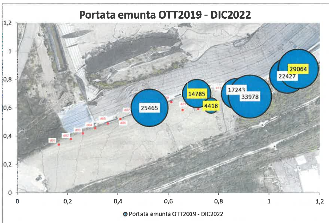
Figura 33 – Rappresentazione grafica delle portate emunte nel periodo OTTOBRE 2019–DICEMBRE 2022 (NB. Le letture in giallo risentono del recente malfunzionamento dei misuratori di portata)
