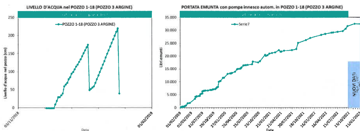
Figura 30 – Portata emunta dal POZZO 1-18 (fino a gennaio 2023)
