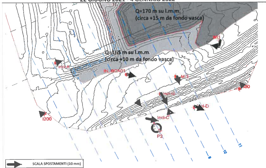
Figura 14 – Spostamenti inclinometrici GEN – GIU 2021 e GIU 2021 – GEN 2022
