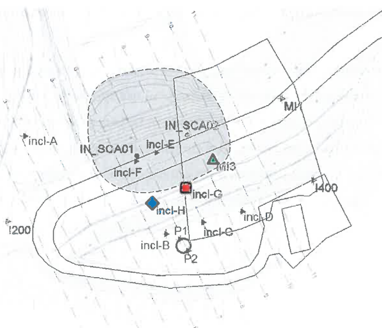
Figura 19 – Inclinometri selezionati per il monitoraggio dell'argine durante il riempimento della discarica
