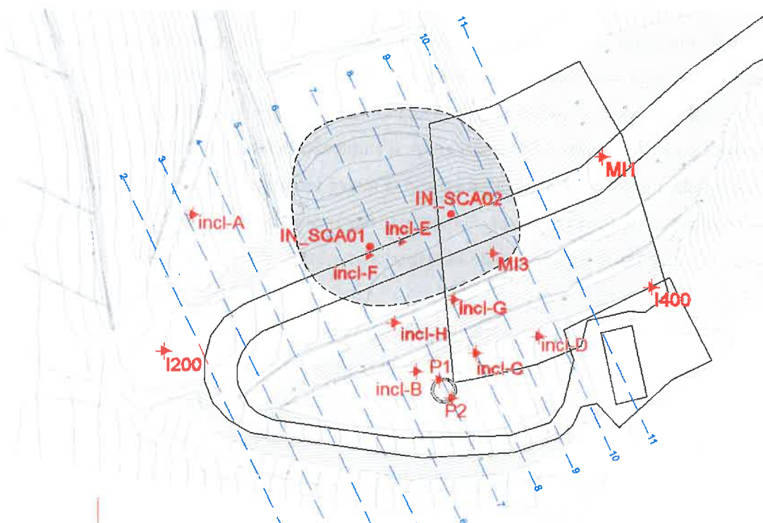
Figura 10 – Planimetria dell'argine con indicazione degli inclinometri operativi a DICEMBRE 2022
