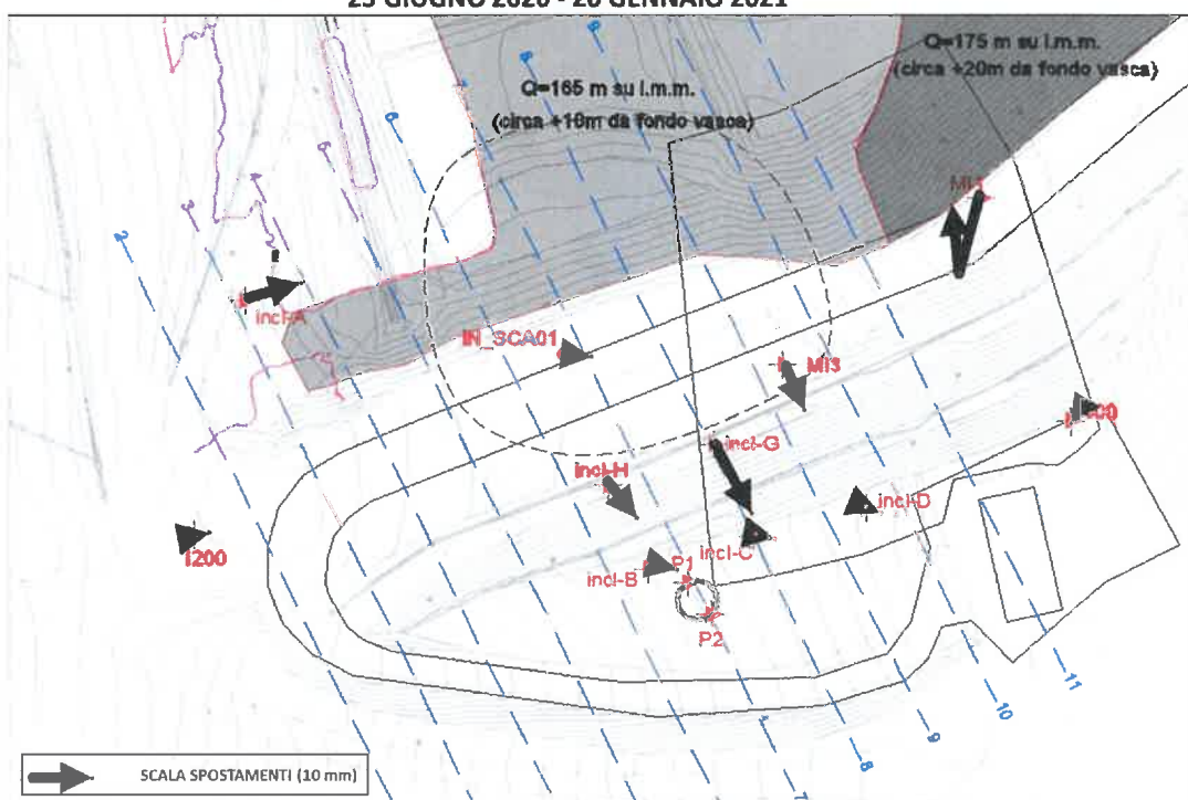
Figura 13 – Spostamenti inclinometrici GEN - GIU 2020 e GIU 2020 - GEN 2021
