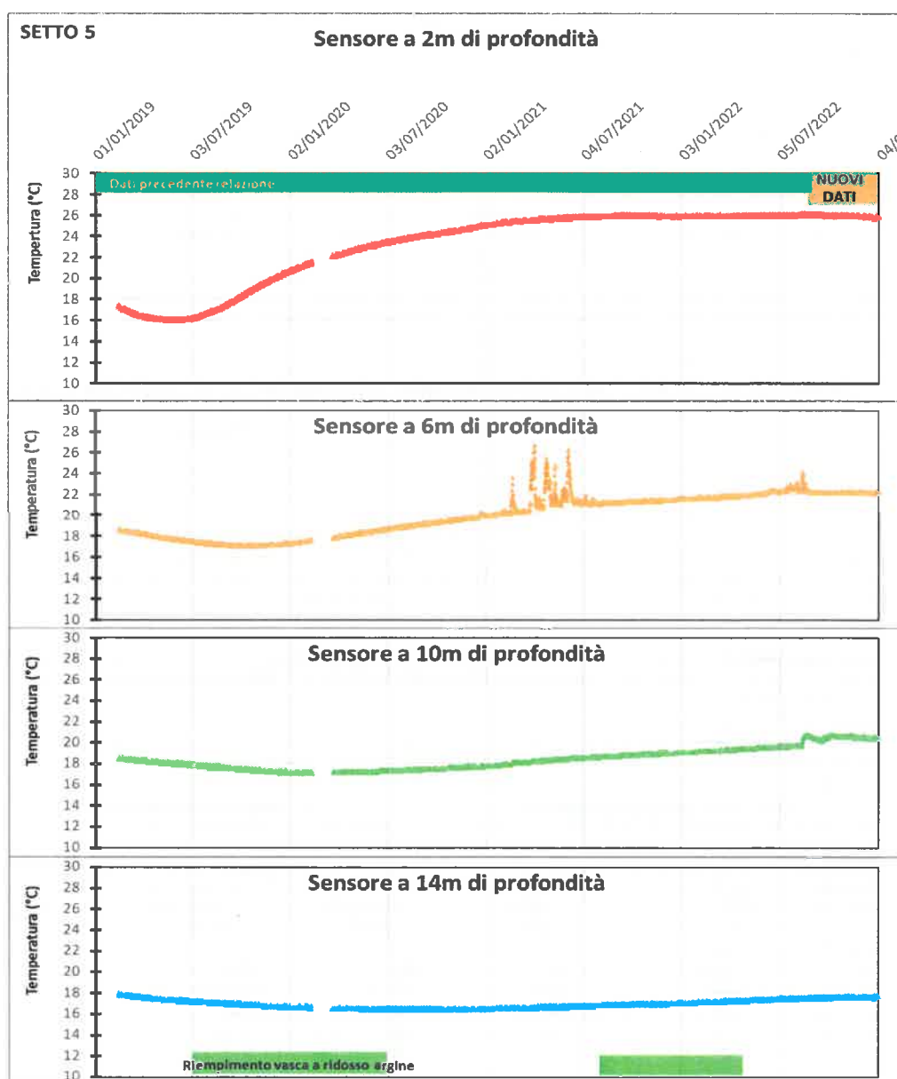
Figura 42 – Andamento temporale della temperatura nei pali D del setto n.5
