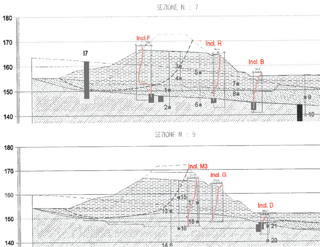
Figura 17 – Forma delle deformate inclinometriche più significative delle sezioni n.7 e n.9 dell'argine
