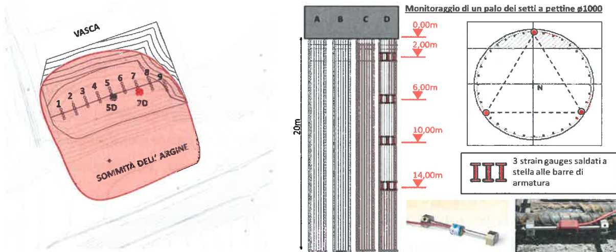
Figura 39 – Posizione dei pali strumentati con strain-gauges e disposizione degli strumenti
