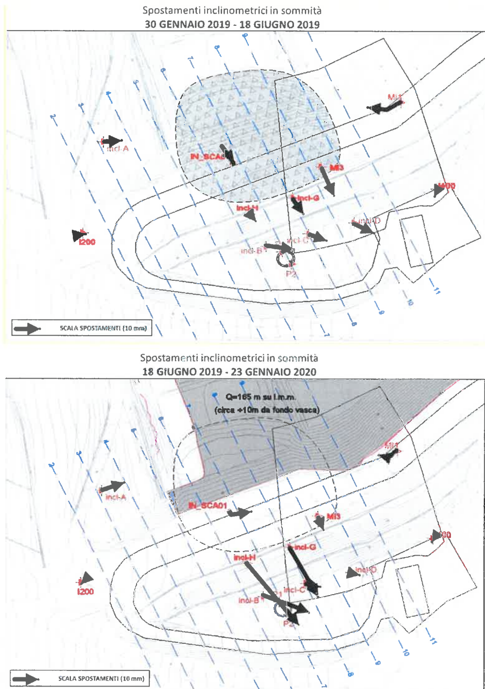
Figura 12 – Spostamenti inclinometrici GEN - GIU 2019 e GIU 2019 – GEN 2020
