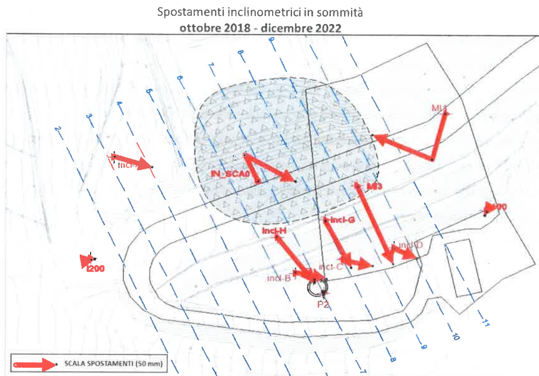
Figura 11 – Spostamenti inclinometrici nel periodo OTTOBRE 2018 – DICEMBRE 2022
