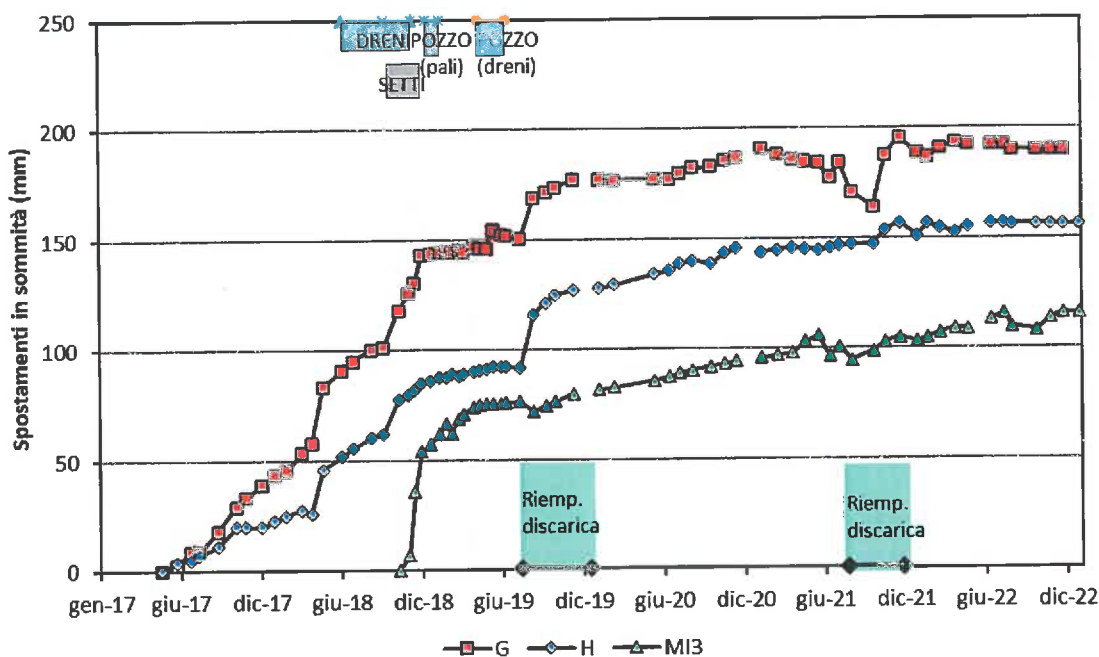
Figura 20 – Andamento nel tempo degli spostamenti in sommità degli Inclinometri G, H e M3
