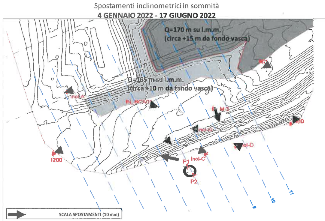
Figura 15 – Spostamenti inclinometrici GEN 2022 – GIU 2022
