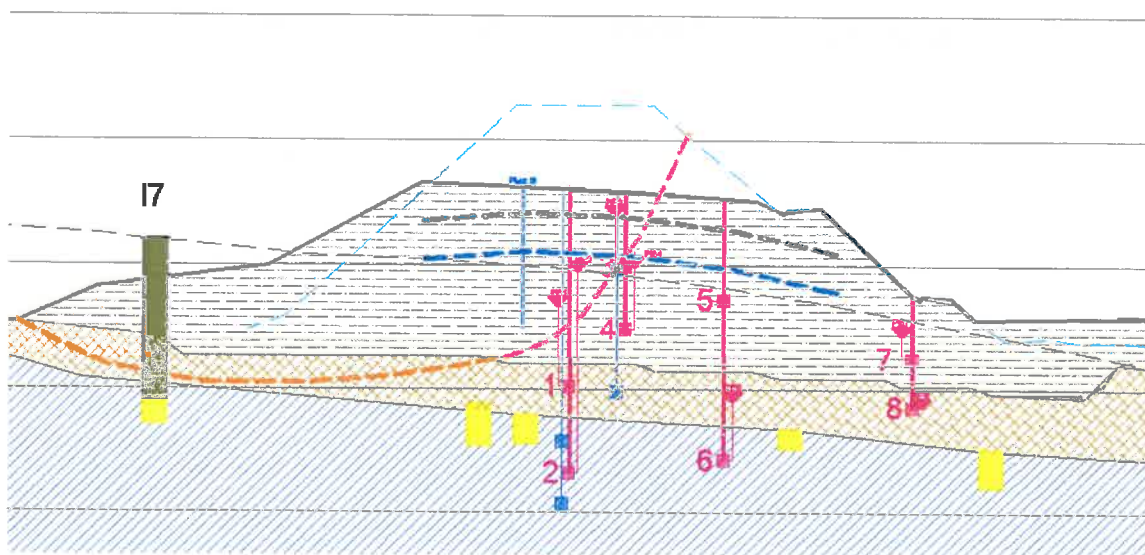
Figura 27 – Confronto tra le altezze piezometriche misurate nel 2018 e nel 2022 nella sezione arginale n.7
