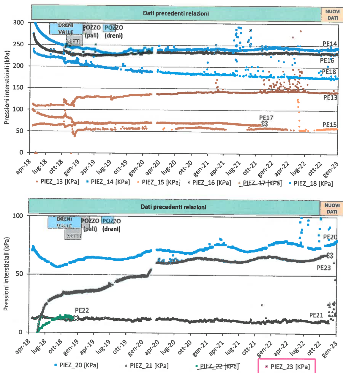
Figura 25 – Andamento nel tempo delle pressioni interstiziali misurate dalle celle PE13-PE23
