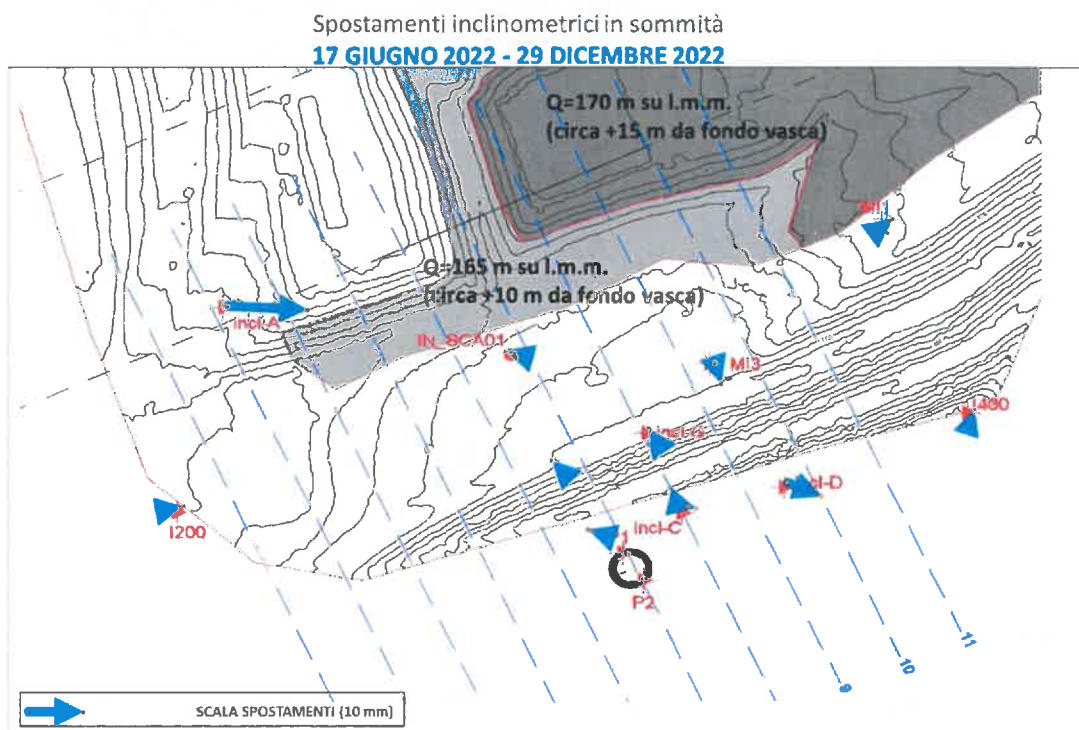
Figura 16 – Spostamenti inclinometrici GIU - DIC 2022
