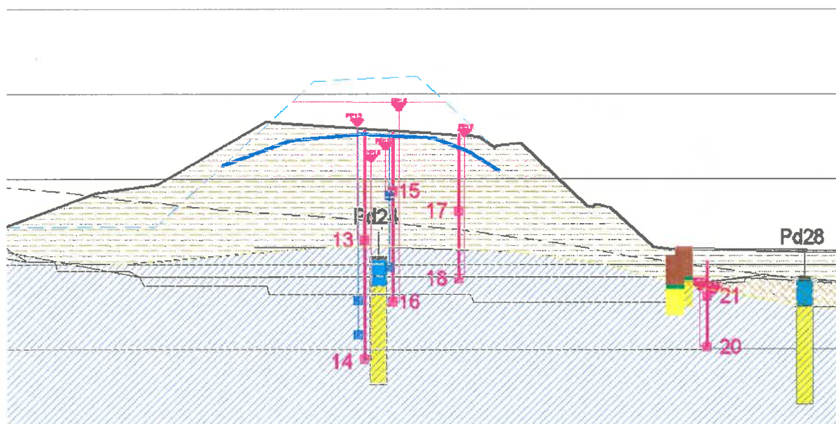
Figura 28 – Confronto tra le altezze piezometriche misurate nel 2018 e nel 2022 nella sezione arginale n.9
