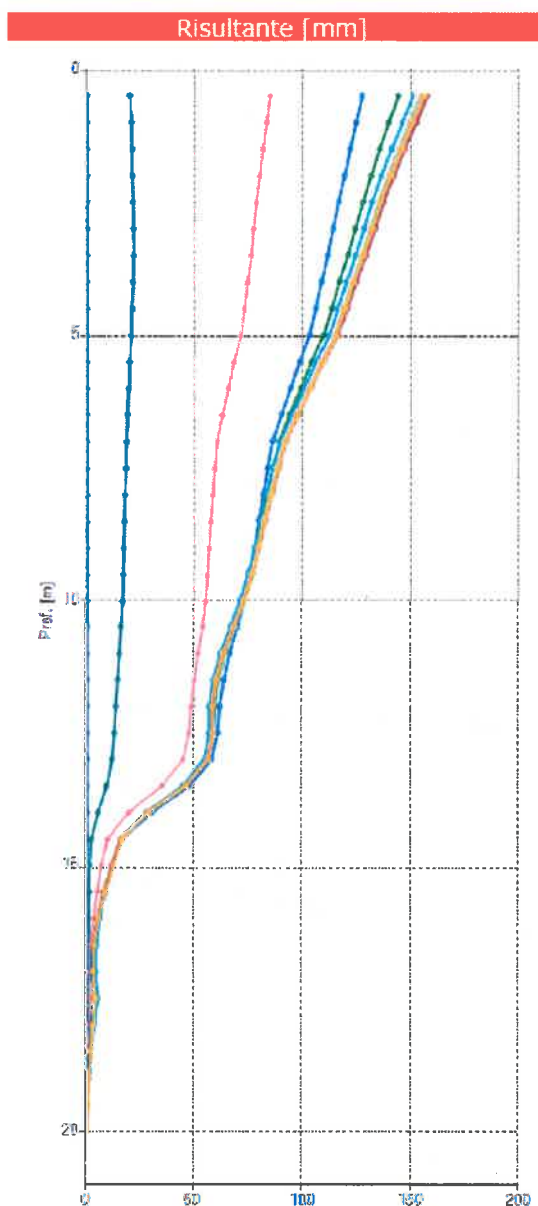
Figura 21 – Inclinometri H (zero al 18-05-2017) e MI3 (zero al 31-10-2018): deformata differenziale integrale dal basso aggiornata al 29-12-2022
